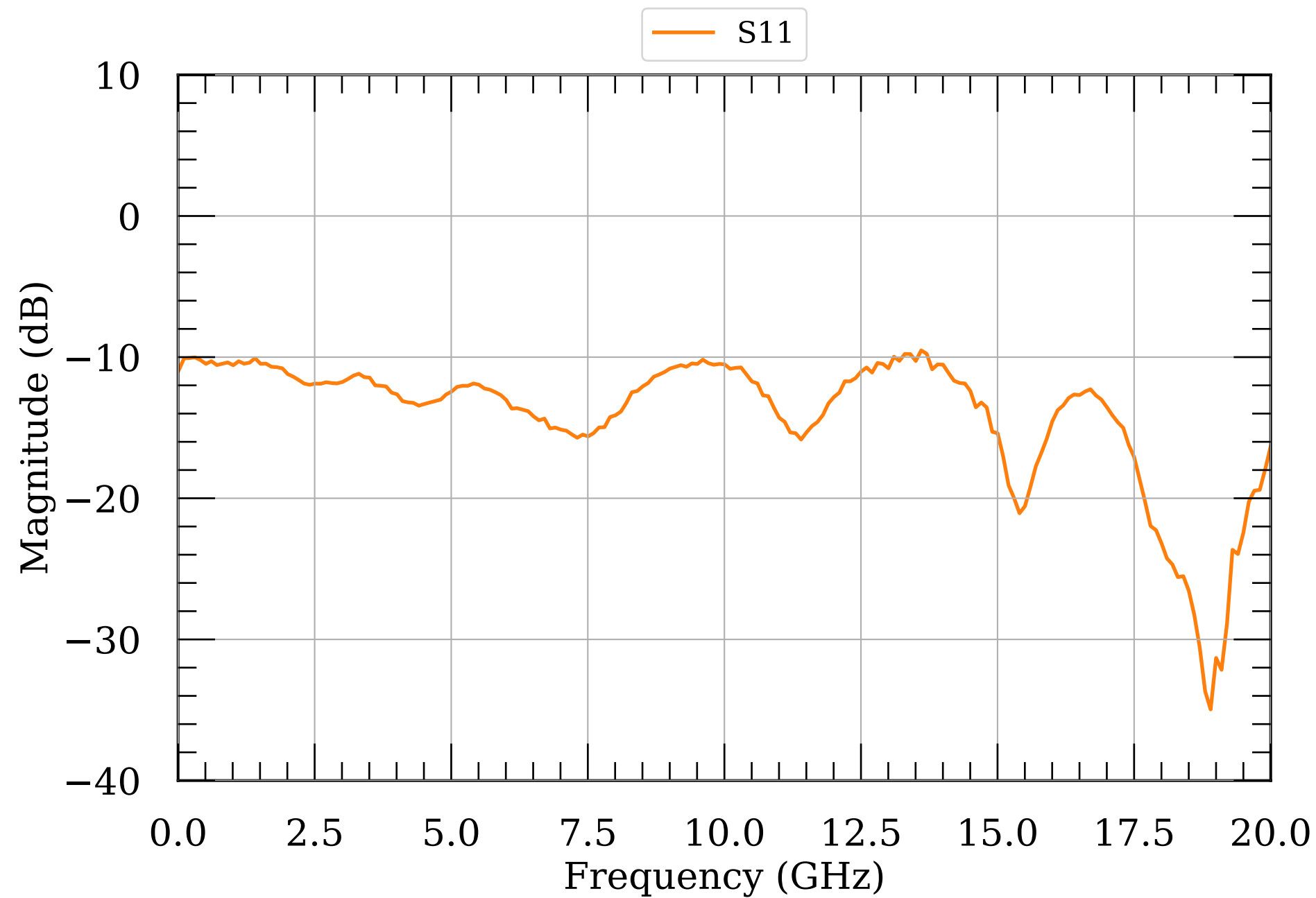
LNA S-params module009
